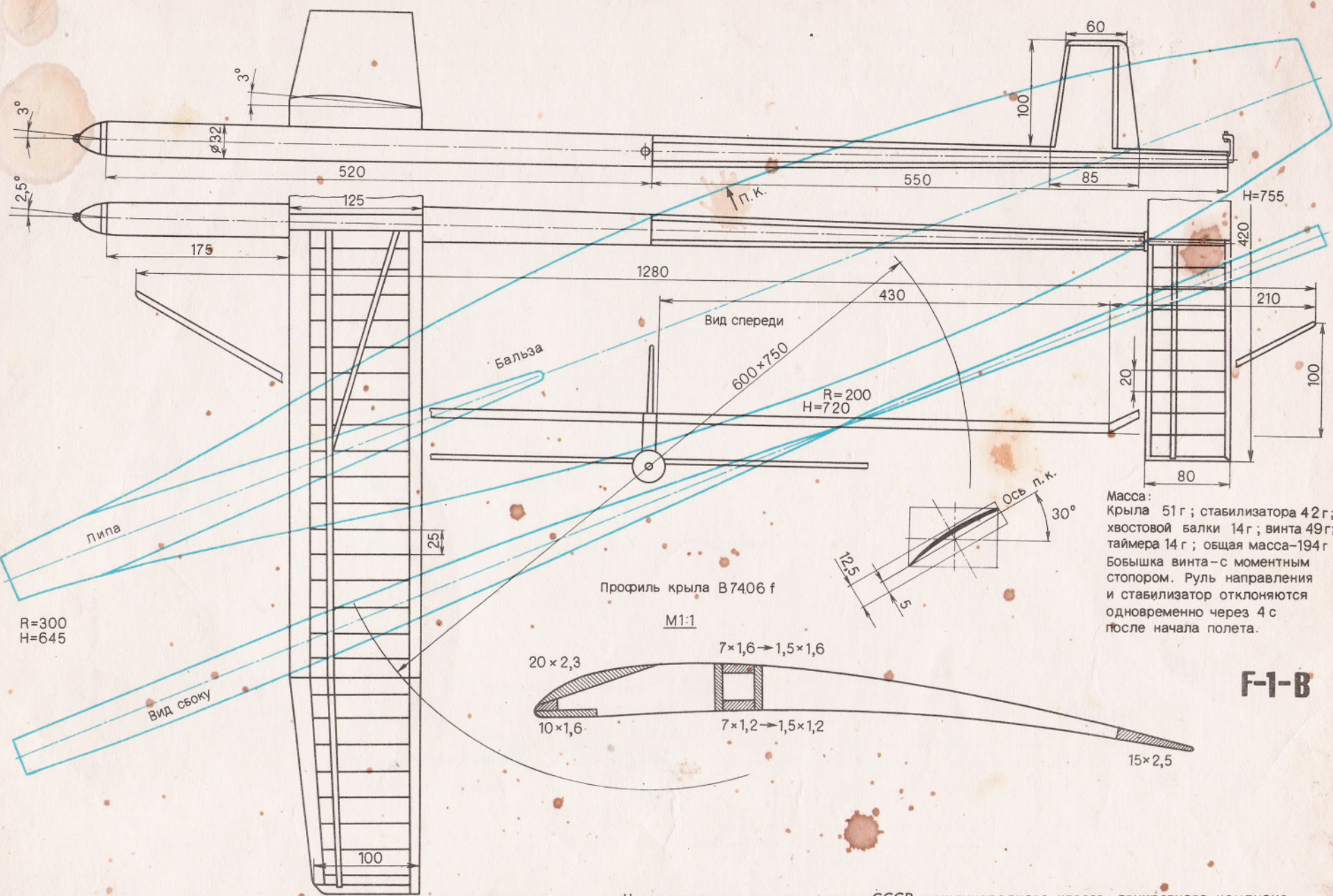
Чертеж модели мастера спорта СССР международного класса, двукратного чемпиона Европы, чемпиона СССР, победителя международных соревнований, члена сборной команды СССР А. Андриюкова (Украина).
