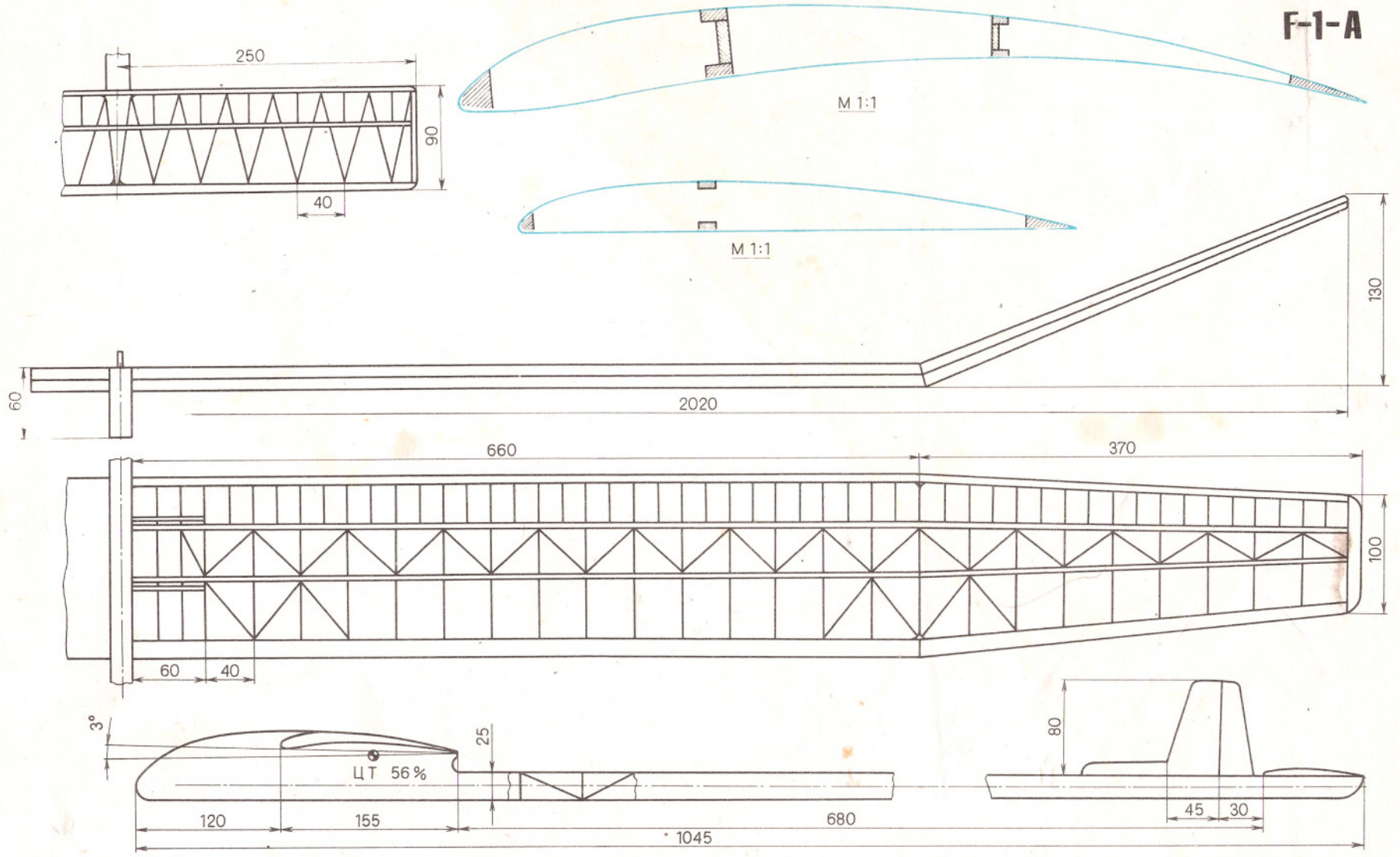
Чертеж модели мастера спорта СССР, чемпиона СССР, члена сборной команды РСФСР И. Кочагова (РСФСР).
