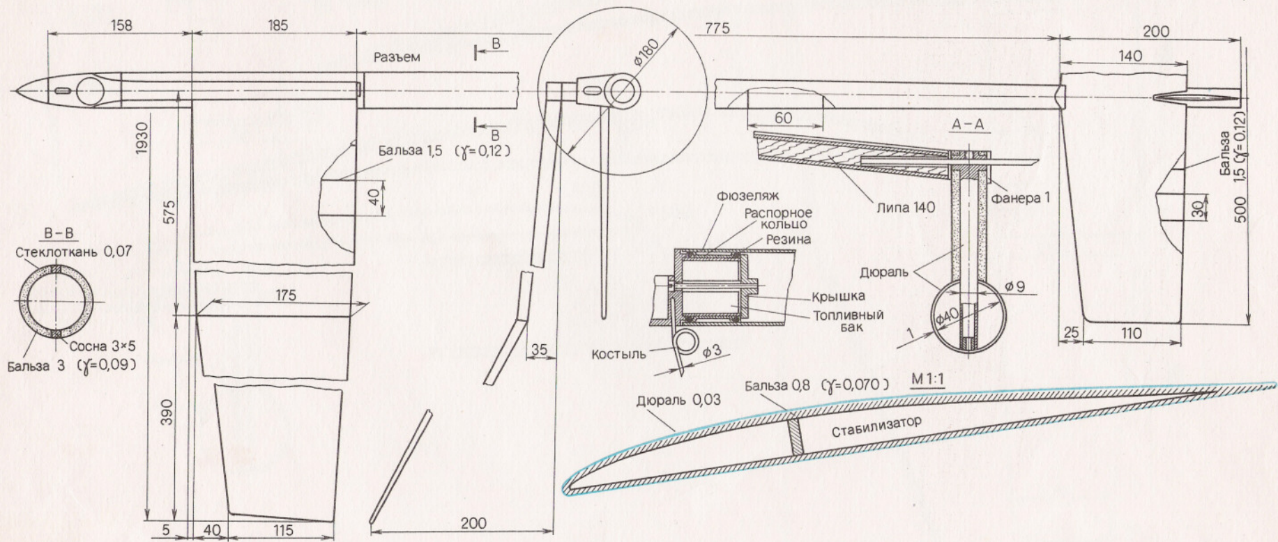
Чертеж модели мастера спорта СССР, призера чемпионата СССР, члена сборной команды Эстонии А. Роотса (Эстония).
