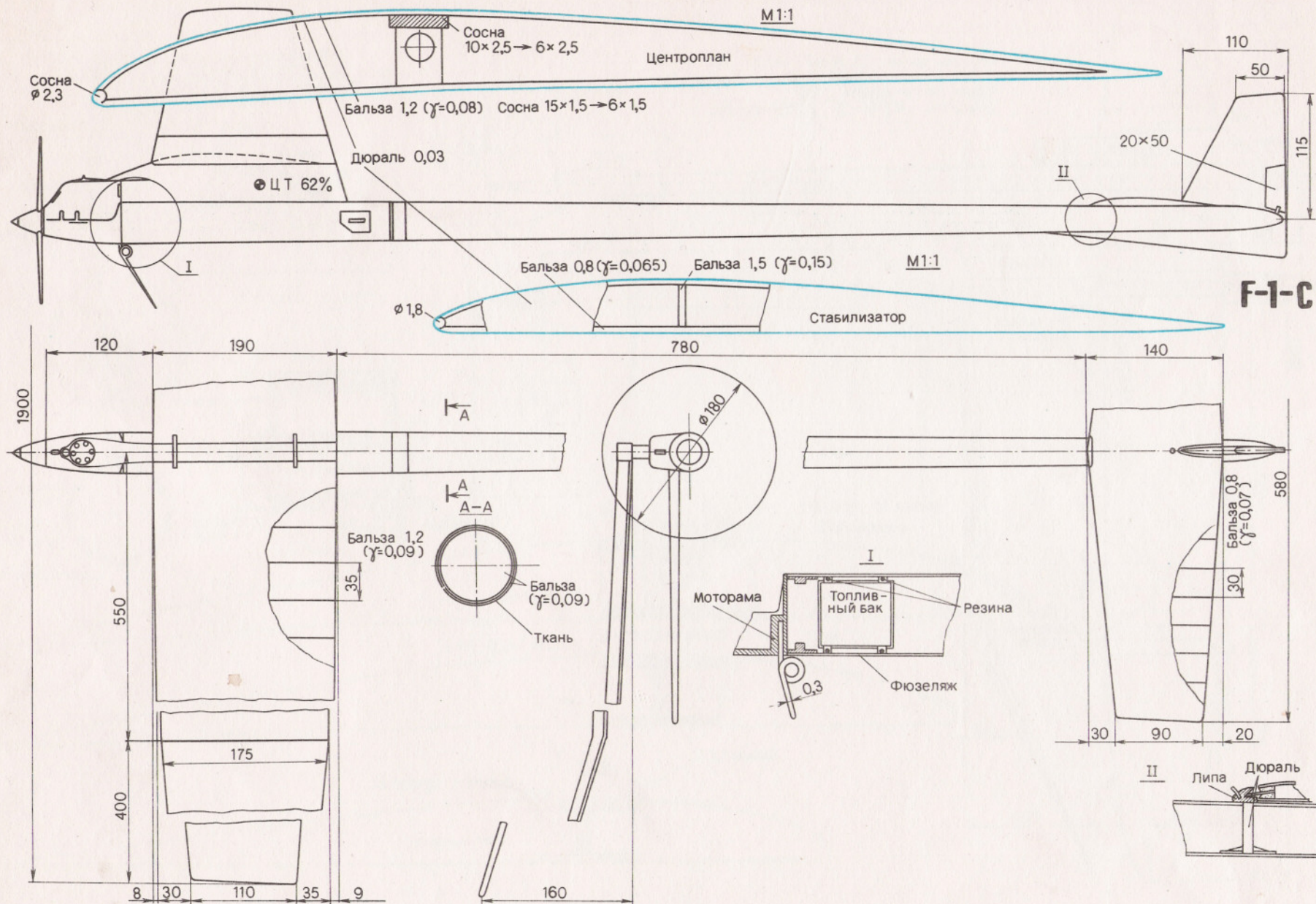
Чертеж модели мастера спорта СССР международного класса, призера чемпиона СССР, члена сборной команды СССР В. Струкова (Украина).
