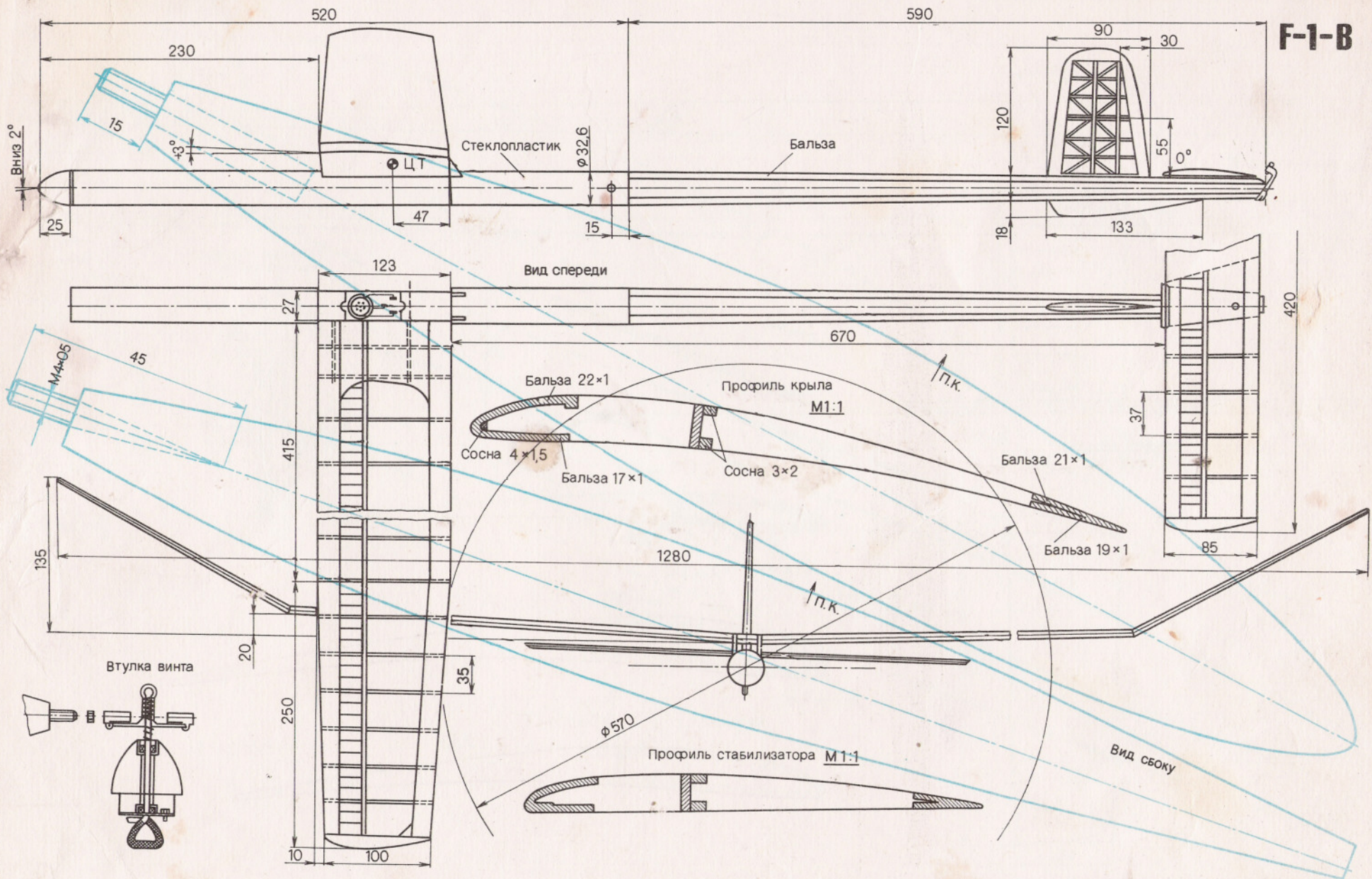
Чертеж модели мастера спорта СССР, призера чемпионата СССР, чемпиона РСФСР, члена сборной команды РСФСР В. Иванова (РСФСР).
