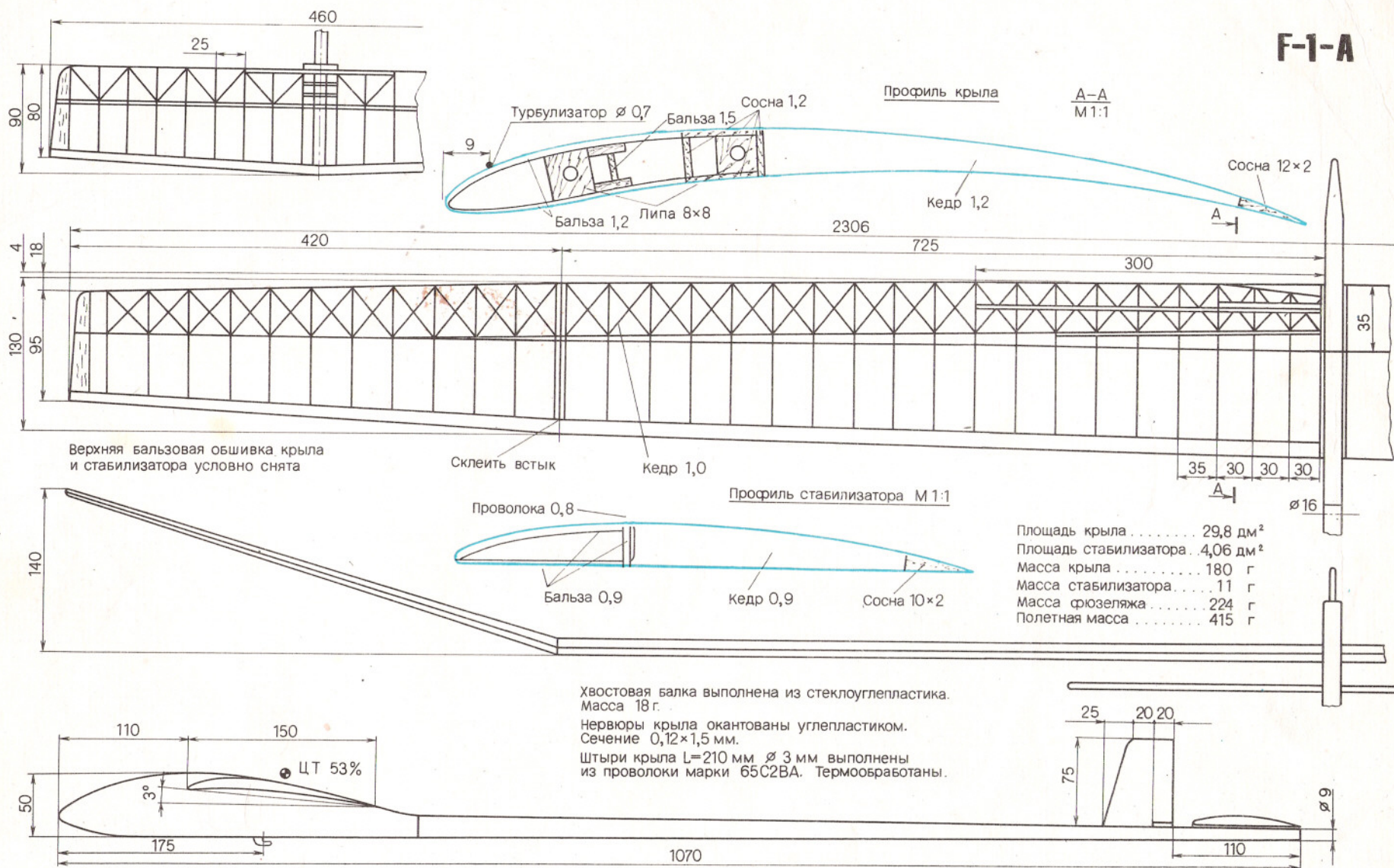
Чертеж модели мастера спорта СССР международного класса, двукратного чемпиона СССР, члена сборной команды СССР Ю. Яблокова (г. Ленинград).
