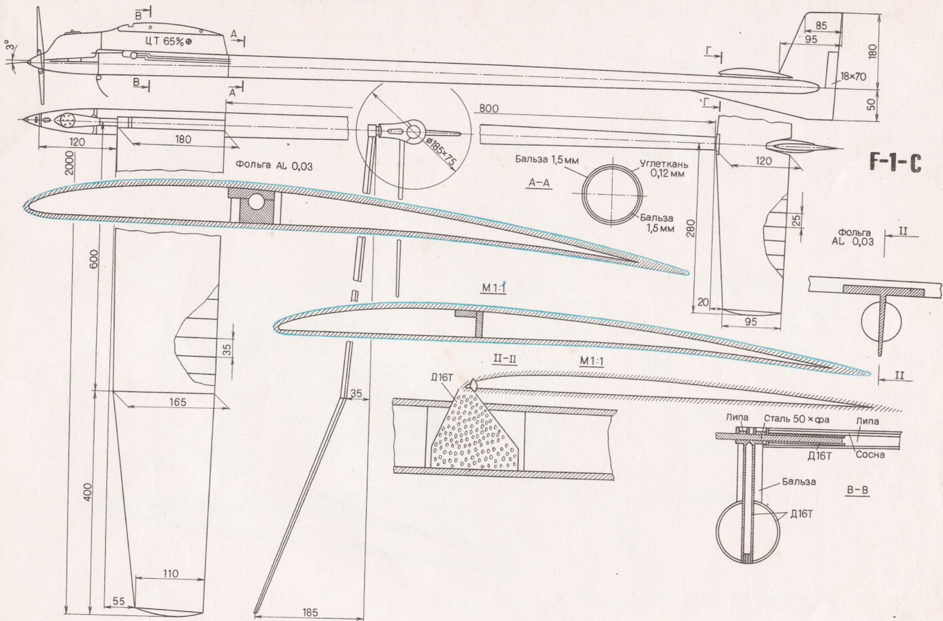
Чертеж модели мастера спорта СССР, чемпиона Европы, СССР, победителя международных соревнований, члена сборной команды СССР Н. Наконечного (Украина).
