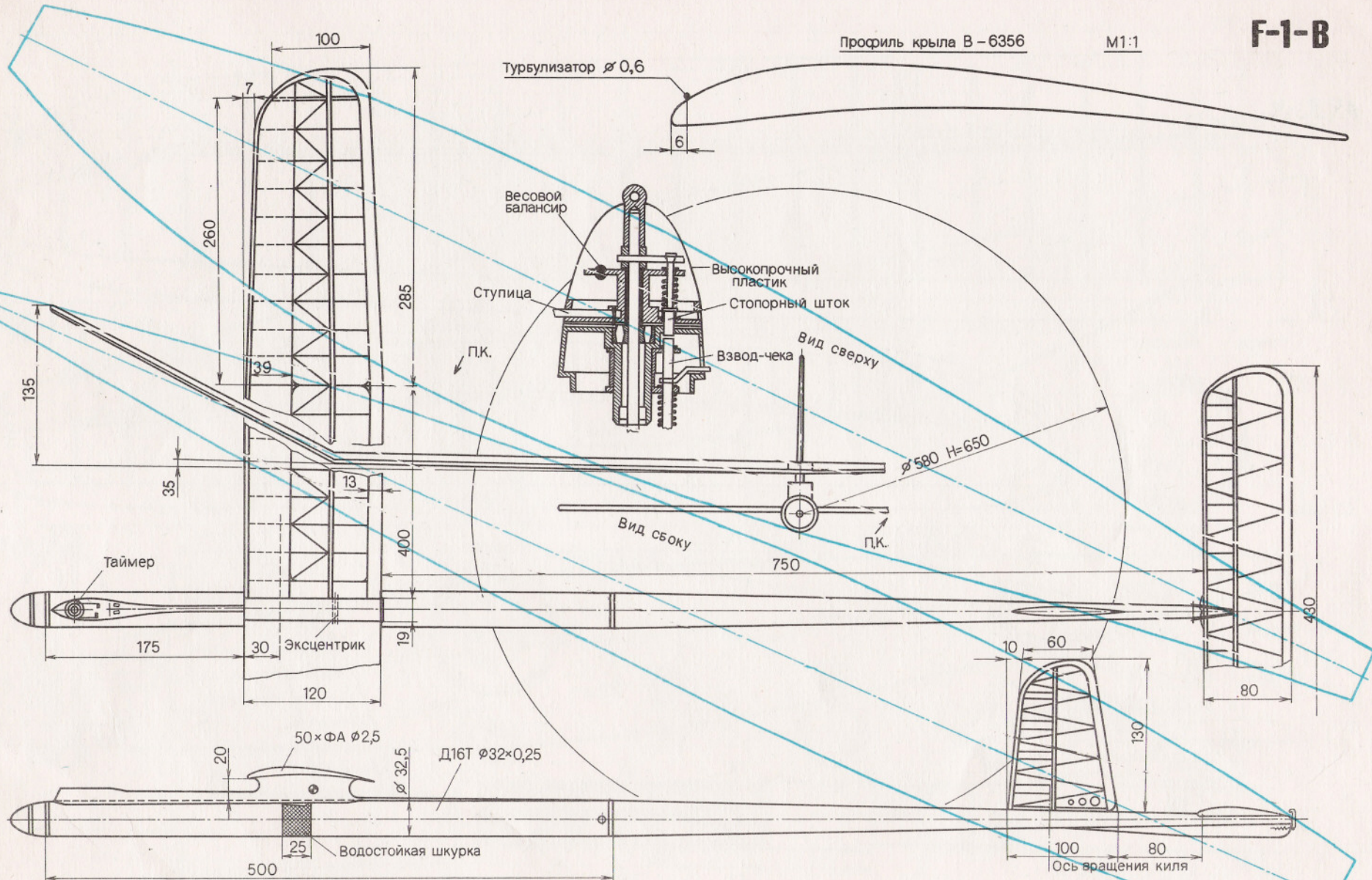
Чертеж модели мастера спорта СССР международного класса, чемпиона СССР, призера чемпионата мира, члена сборной команды СССР С. Самокиша (Украина).
