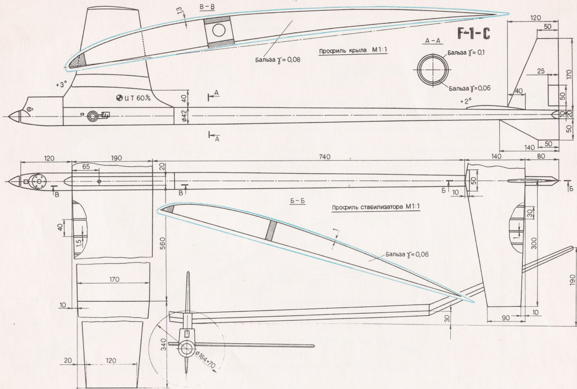
Чертеж модели мастера спорта СССР, чемпиона СССР, члена сборной команды г. Москвы Н. Шкаликова (г. Москва).
