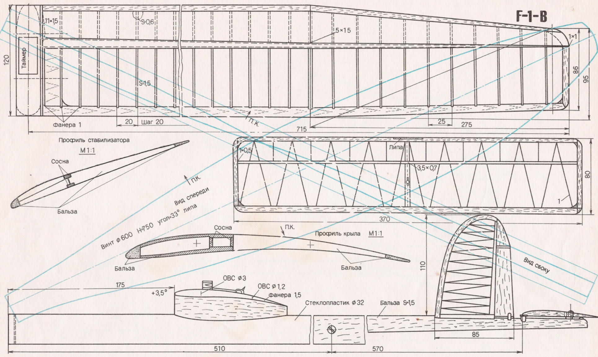
Чертеж модели мастера спорта СССР, чемпиона РСФСР Ю. Усова (РСФСР).
